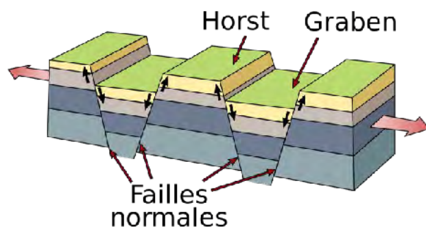
Schéma d'une succession de horst/graben (source wikipédia).
